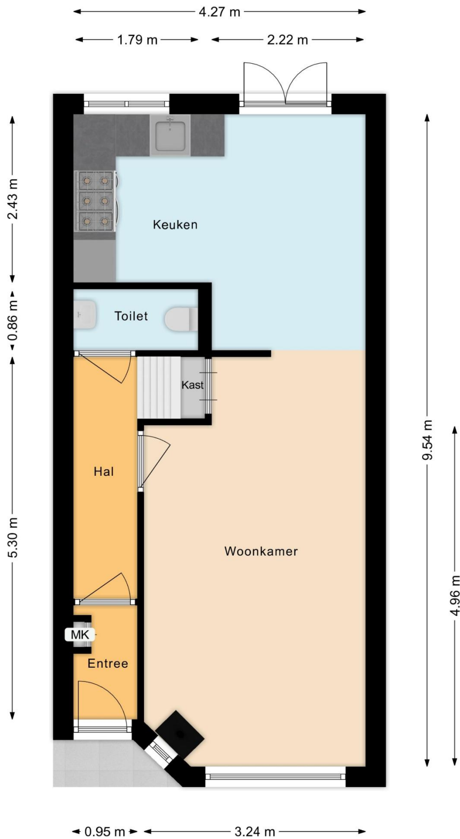
Eerste woonlaag, Loenensestraat 75 te Den Haag
