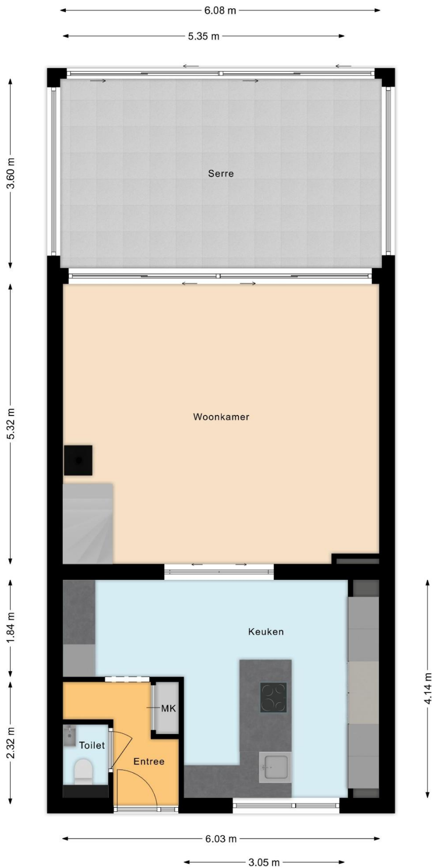
Eerste woonlaag, Zandkamp 8 te Hoogland
