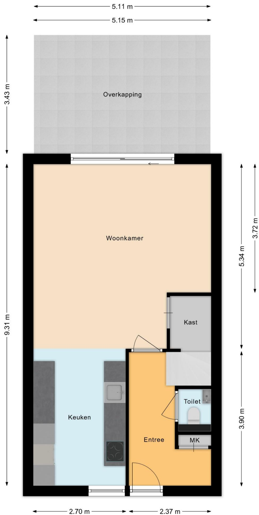
Eerste woonlaag, Tournooiruwe 31 te Maastricht
