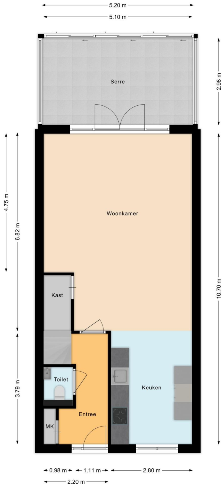
Eerste woonlaag, Kiekendief 17 te Lichtenvoorde
